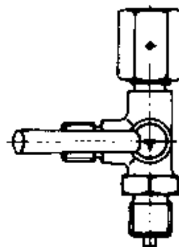
ISPUST DOVOD OTVOREN MANOMETAR IZVAN POGONA TLAČNI MEDIJ SLOBODNO IZLAZI
