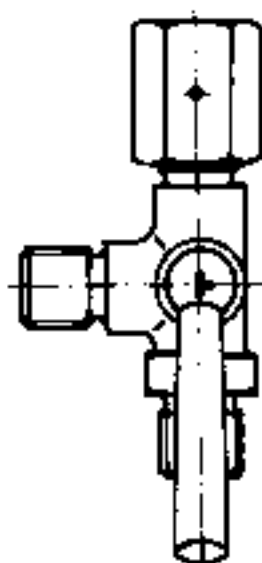
POGON DOVOD OTVOREN MANOMETAR POD TLAKOM
