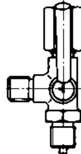
ISPITIVANJE DOVOD OTVOREN MANOMETAR I PROBNI INSTRUMENT POD TLAKOM
