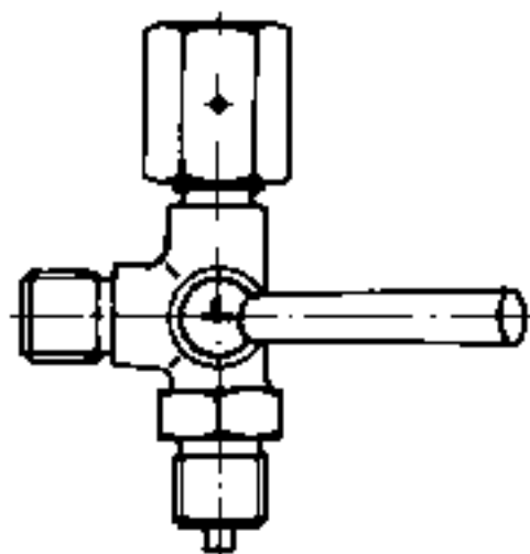
ODZRAČIVANJE DOVOD ZATVOREN NULTA POZICIJA
